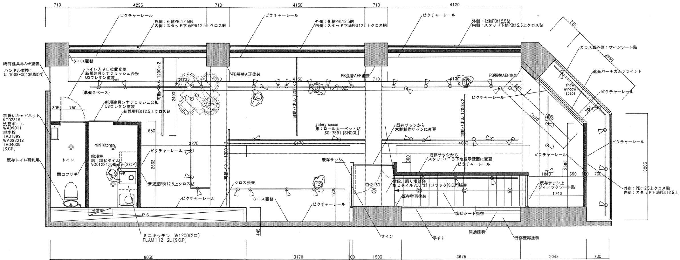
平面図
